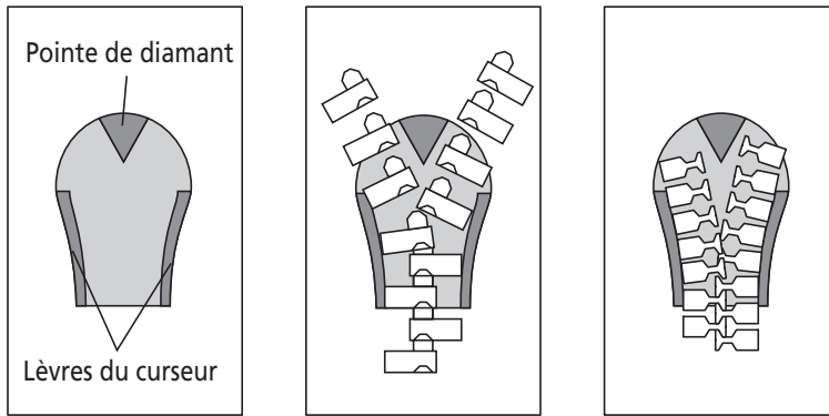
Figure 1.3 La fermeture éclair
