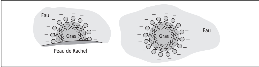
Figure 8.8 L'action des molécules de savon sur les graisses
