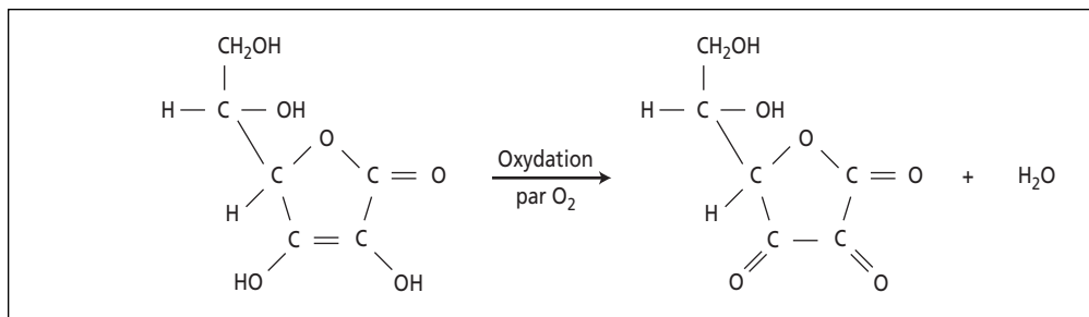
Figure 7.6 L'oxydation de la vitamine C
