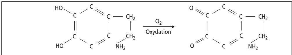
Figure 7.5 Oxydation d'un composé phénolique
