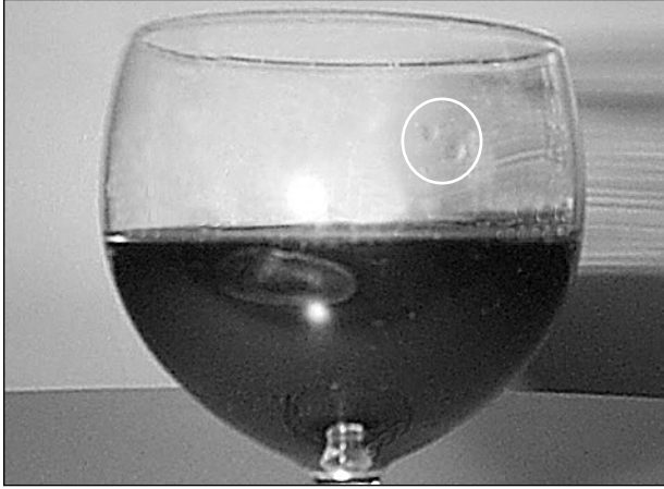
Figure 7.3 Les larmes du vin
