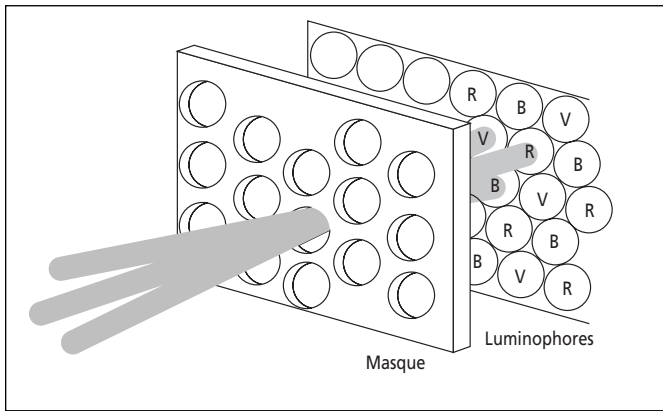
Figure 9.3 Masque et luminophores de la télé couleur
