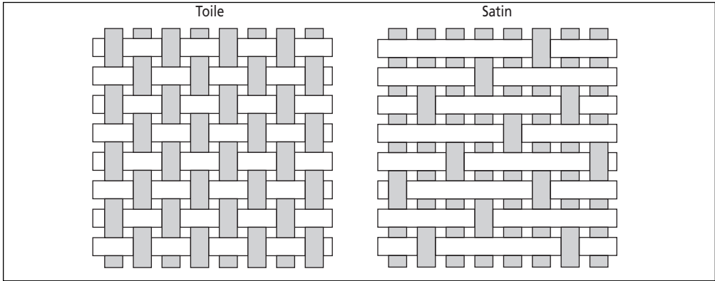
Figure 1.2 Deux types d'armures pour les tissus
