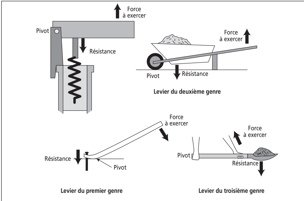
Figure 7.2 Différents genres de leviers
