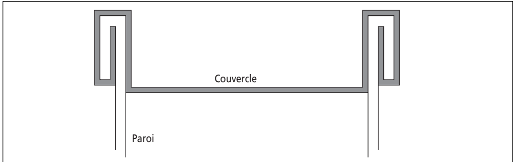
Figure 4.2 Coupe transversale d'une boîte de conserve
