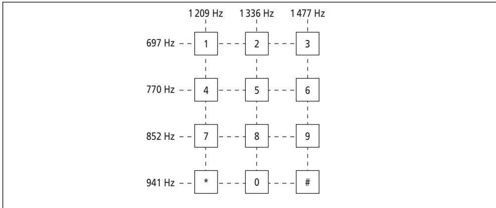
Figure 5.1 Clavier de téléphone et fréquences émises lorsqu'on appuie sur un bouton
