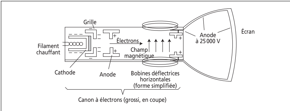
Figure 9.2 Schéma en coupe d'un canon à électrons
