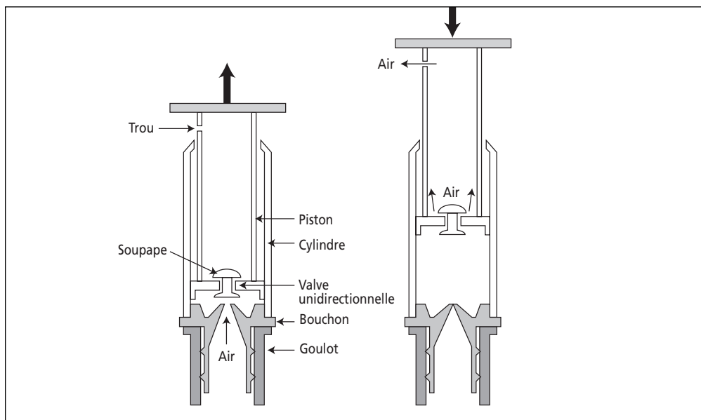
Figure 8.2 Bouchon et pompe de type Vacu-Vin vus en coupe
