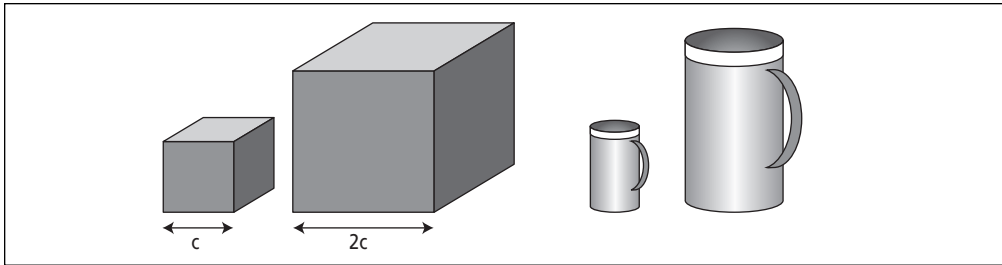
Figure 2.2 Effet du rapport surface-volume
