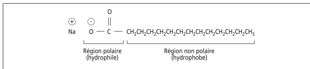
Figure 8.6 Une molécule de savon typique: le myristate de sodium (CH 3 (CH 2 ) 12 COONa)
