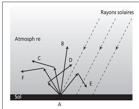
Figure 3.1 Transferts d'énergie à la surface de la Terre
