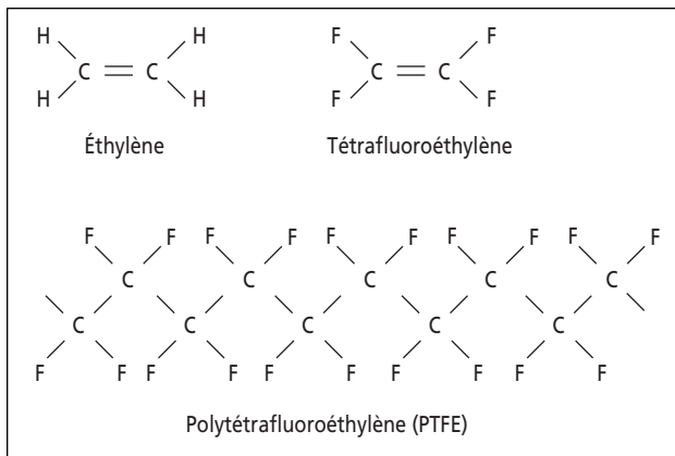
Figure 6.2 Structures chimiques de l'éthylène, du tétrafluoroéthylène et du téflon ®
