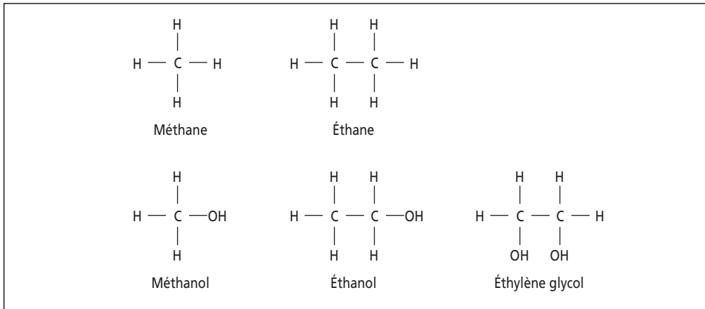
Figure 7.1 Structure de quelques composés organiques
