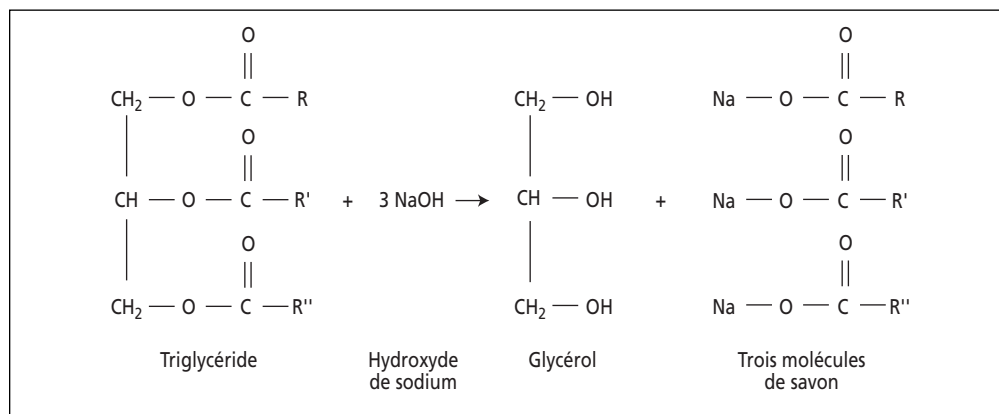
Figure 8.5 Réaction de fabrication du savon
