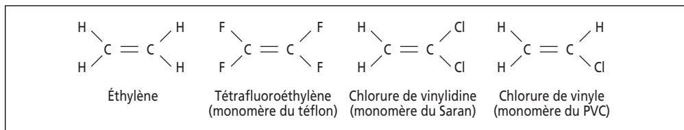
Figure 8.1 Structures chimiques de l'éthylène, du tétrafluoroéthylène, du chlorure de vinylidène et du chlorure de vinyle
