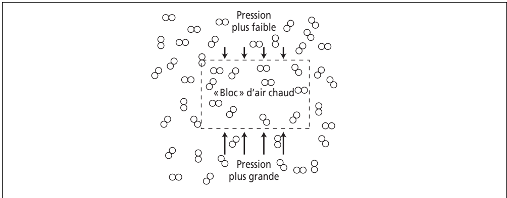
Figure 6.3 Force d'Archimède dans l'air
