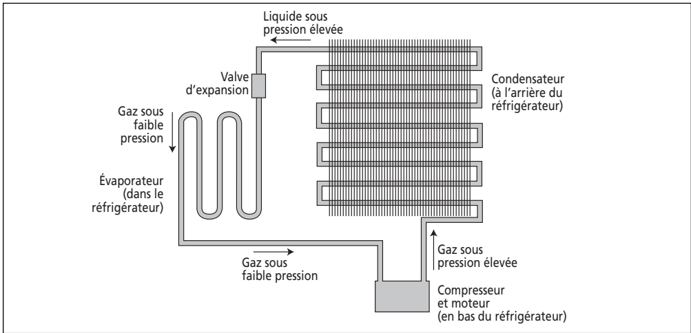
Figure 6.1 Cycle du fluide de réfrigération
