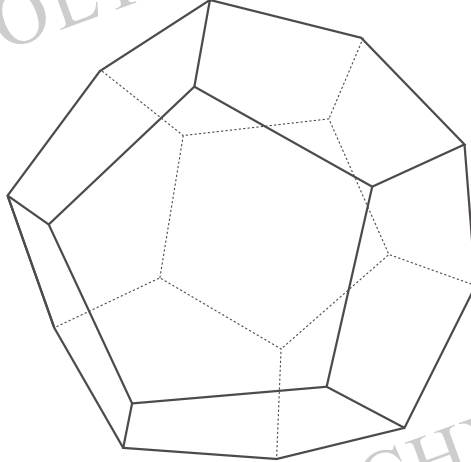
FIG. 3. Le dodécaèdre
